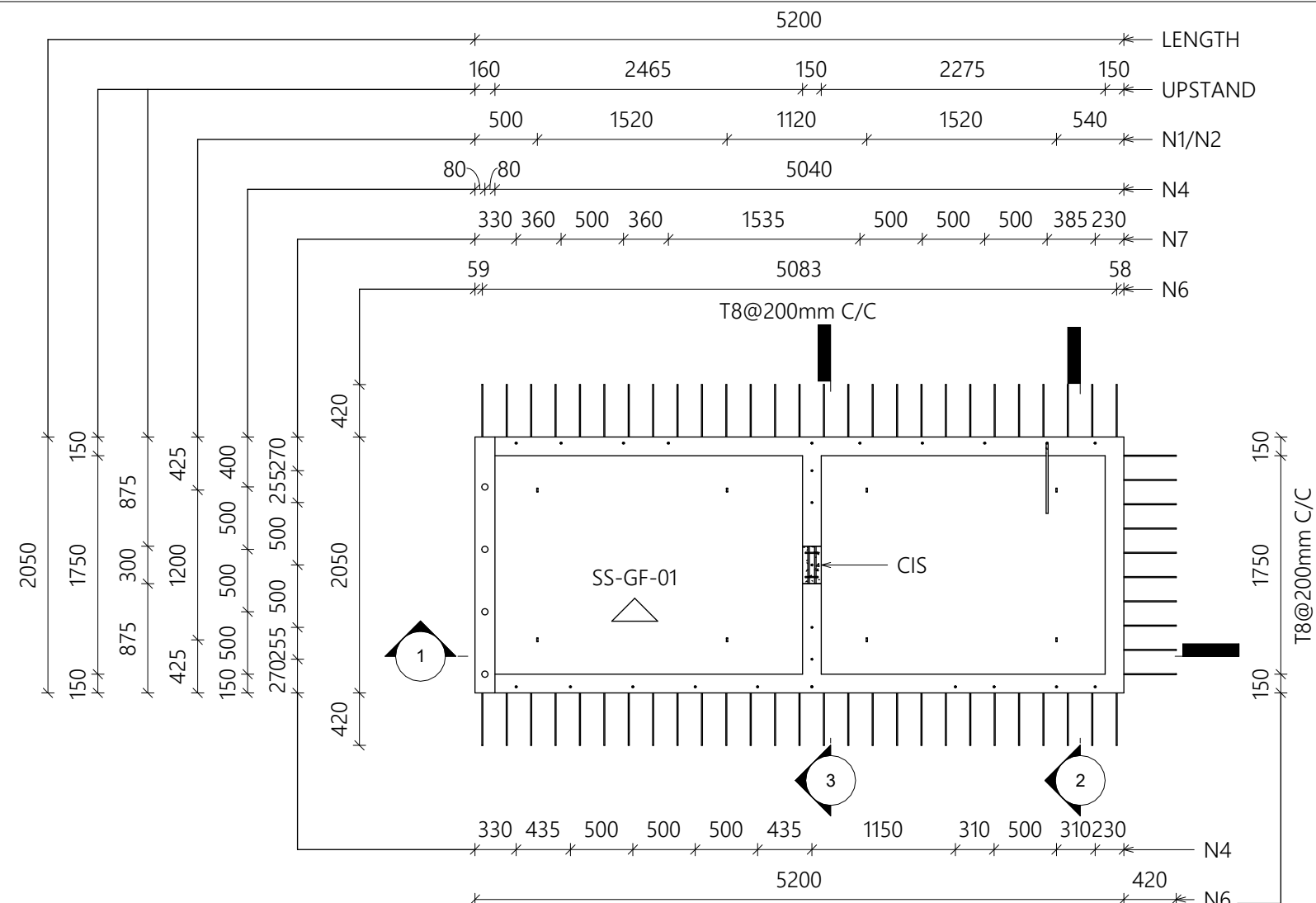
A TOP PLAN 1 : 50
